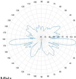
3860 MHz
