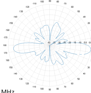
2320 MHz
