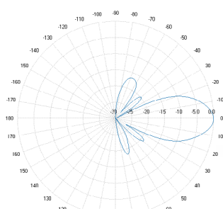
2620 MHz
