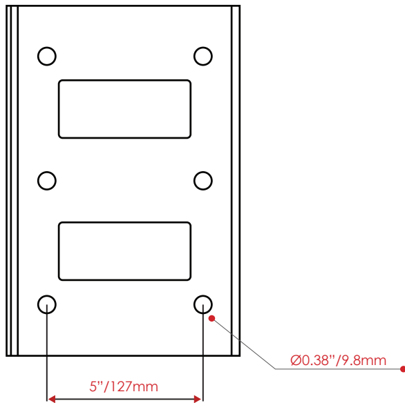
Extension Module.
