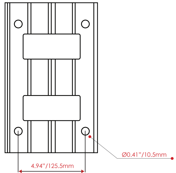
Tilt Module.
